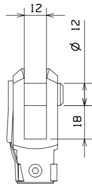
DETAIL BELIERE ECHELLE 1:2
