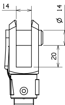
Detail beliere Echelle 1:2
