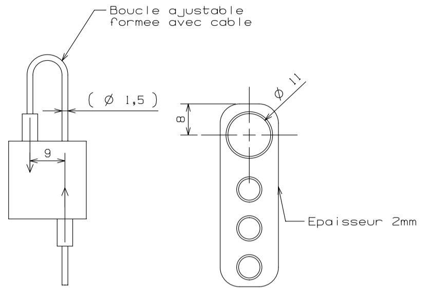
Detail systeme de fixation Ech 1:1
